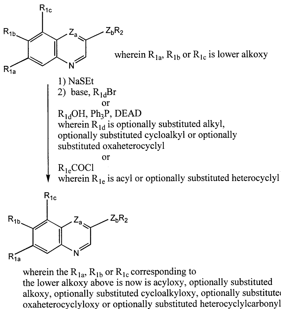
Scheme VI
