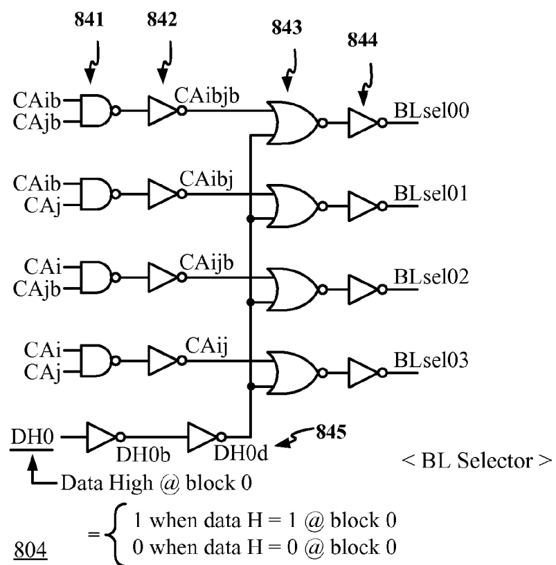
FIG. 10A
