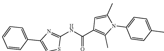
2,5-dimethyl-N-(4-phenylthiazol-2-yl)-1-(p-tolyl)-1H-pyrrole-3-carboxamide (16)
