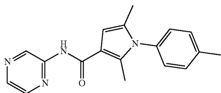
2,5-Dimethyl-N-(pyrazin-2-yl)-1-(p-tolyl)-1H-pyrrole-3-carboxamide (15)
