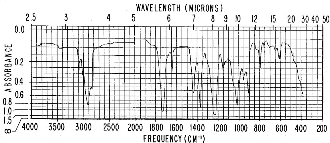
IR SPECTRUM FOR EXAMPLE XXXIV.
