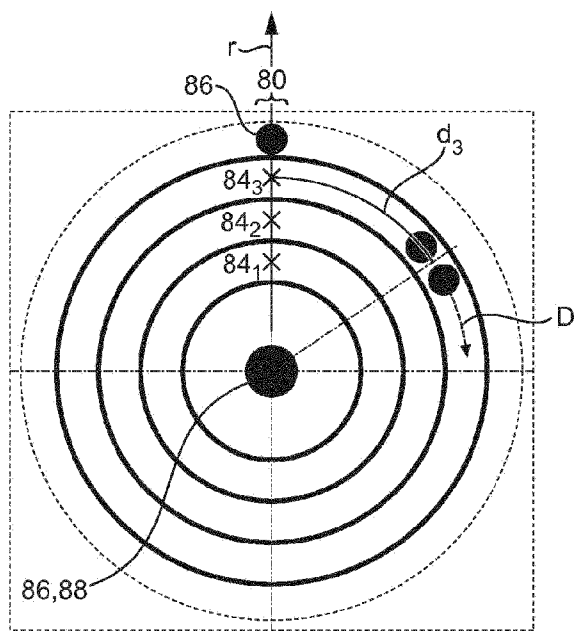
FIG. 5D
