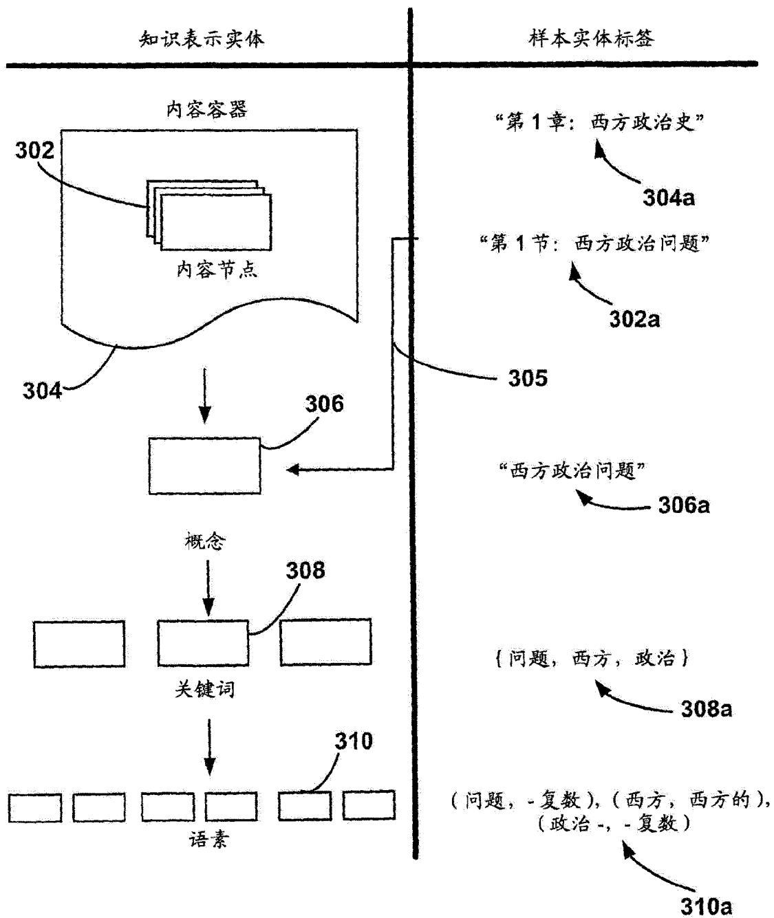
知识表示模型
