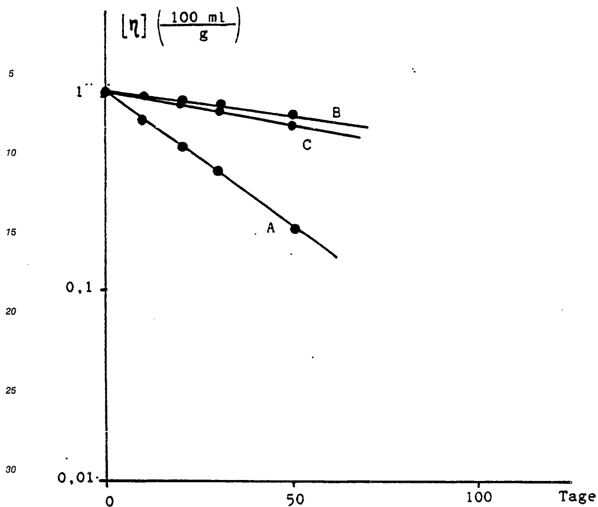
Abb. 1: Molmassenabnahme von Polylaktid-Implantaten
