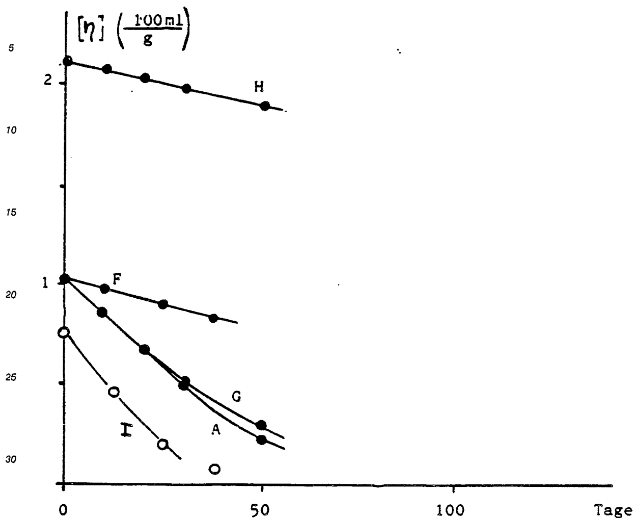
Abb. 5 Molmassenabnahme von Polylaktid-Implantaten
