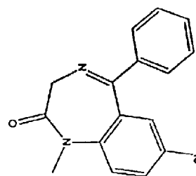
Diazepam (Valium) - Site II
