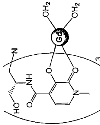
Gd(SerTREN-1-Me-HOPO)(H 2 O) 2
