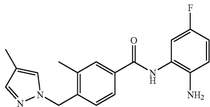
N-(2-amino-5-fluorophenyl)-3-methyl-4- ((4-methyl-1H-pyrazol-1-yl)methyl)benzamide
