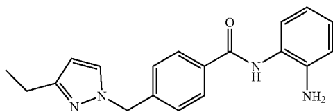
N-(2-aminophenyl)-4-((3-ethyl-1H-pyrazol-1- yl)methyl)benzamide
