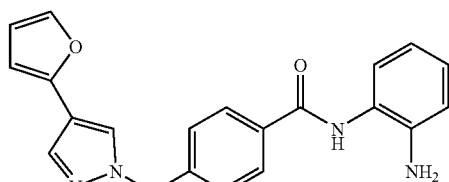
N-(2-aminophenyl)-4-((4-(furan-2-yl)-1H- pyrazol-1-yl)methyl)benzamide
