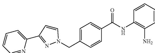
N-(2-aminophenyl)-4-((3-(pyridin-2-yl)-1H-pyrazol-1-yl)methyl)benzamide
