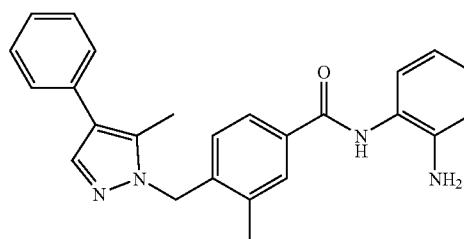
N-(2-aminophenyl)-3-methyl-4-((5-methyl- 4-phenyl-1H-pyrazol-1-yl)methyl)benzamide
