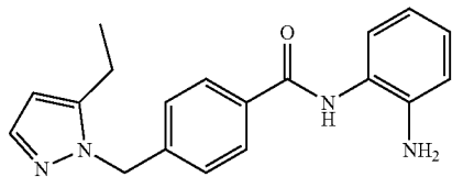
N-(2-aminophenyl)-4-((5-ethyl-1H-pyrazol- 1-yl)methyl)benzamide
