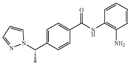
(S)-4-(1-(1H-pyrazol-1-yl)ethyl)-N-(2-aminophenyl)benzamide
