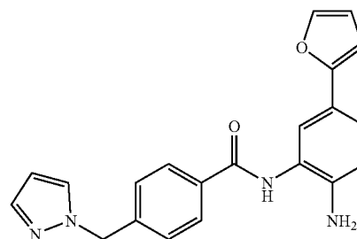
4-((1H-pyrazol-1-yl)methyl)-N-(2-amino-5- (furan-2-yl)phenyl)benzamide
