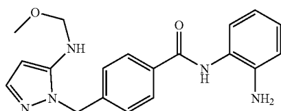
N-(2-aminophenyl)-4-((5-(methoxymethylamino)-1H-pyrazol-1-yl)methyl)benzamide
