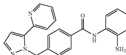
N-(2-aminophenyl)-4-((5-(pyridin-2-yl)-1H- pyrazol-1-yl)methyl)benzamide
