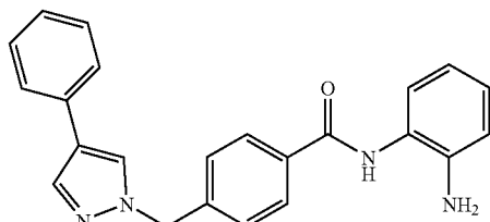
N-(2-aminophenyl)-4-((4-phenyl-1H-pyrazol- 1-yl)methyl)benzamide
