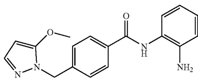
N-(2-aminophenyl)-4-((3-methoxy-1H-pyrazol-1-yl)methyl)benzamide
