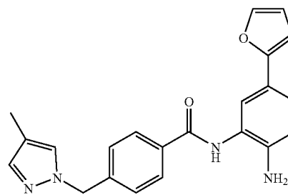
N-(2-amino-5-(furan-2-yl)phenyl)-4-((4- methyl-1H-pyrazol-1-yl)methyl)benzamide
