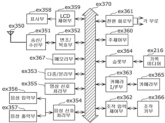
도면25
