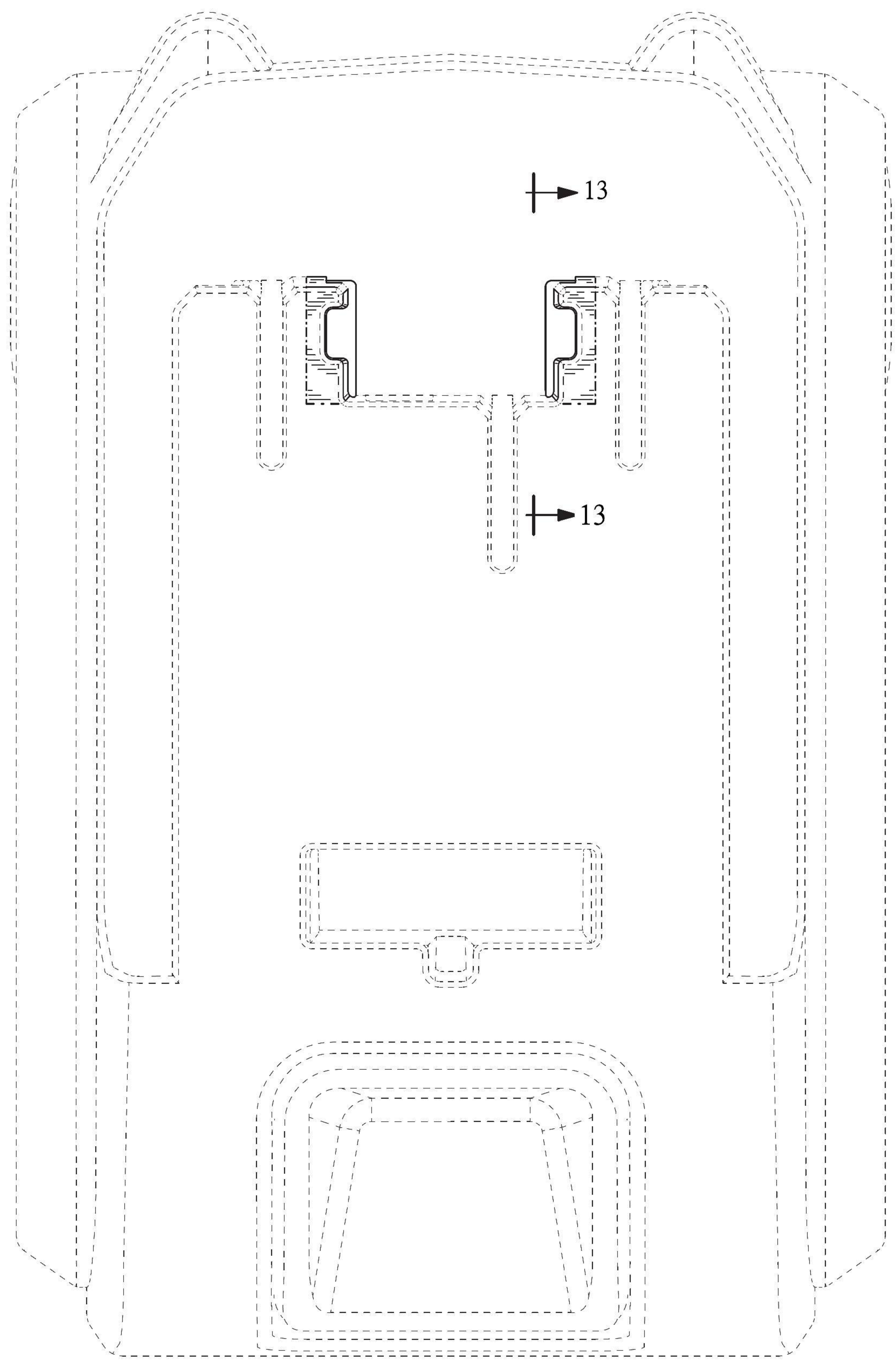
【俯視圖】
