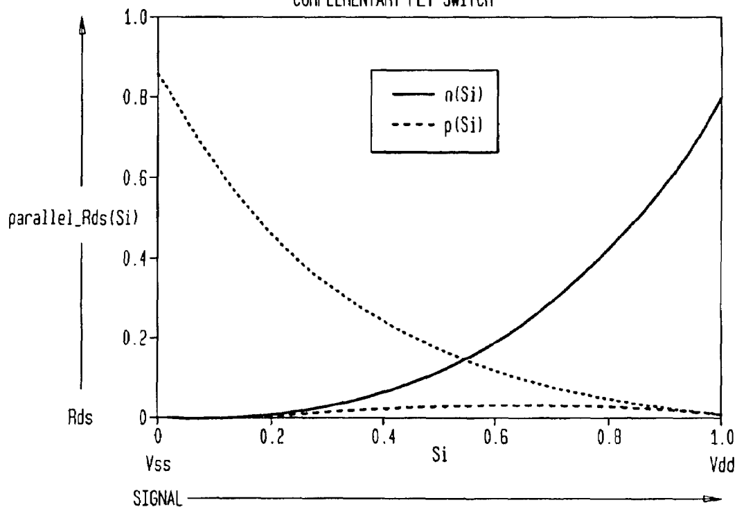
FIG. 241 COMPLEMENTARY FET SWITCH
