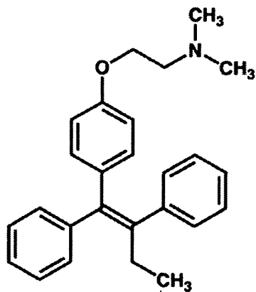
Erlotinib
