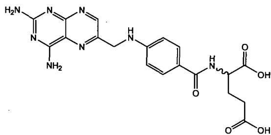
Aminopterin
