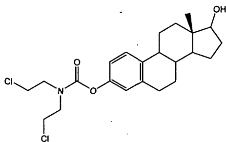
Estramustine
