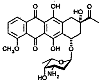
Daunorubicin
