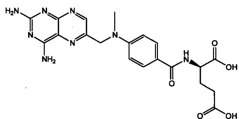
Methotrexate
