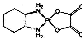
Oxaliplatin
