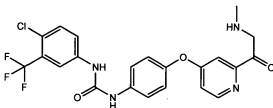
Sorafenib
