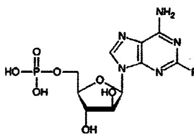
Fludarabine
