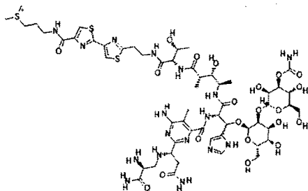
Bleomycin
