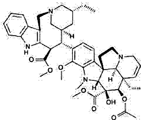
Vinorelbine
