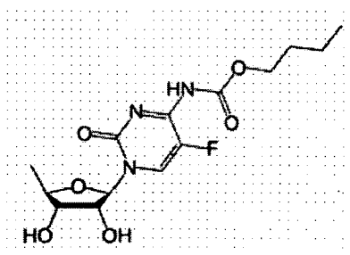
Capecitabine
