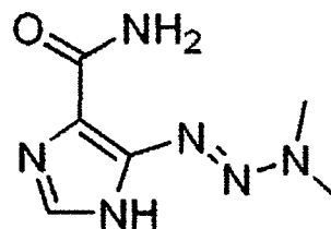
Dacarbazine
