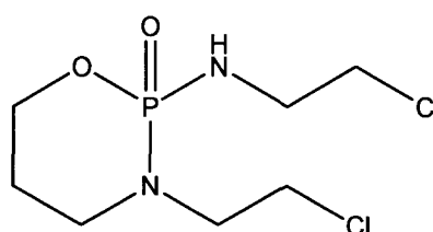
Ifosfamide
