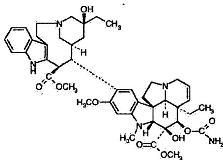
Vindesine
