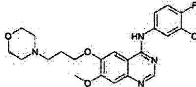
Gefitinib
