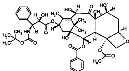
Docetaxel
