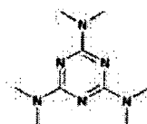
Altretamine
