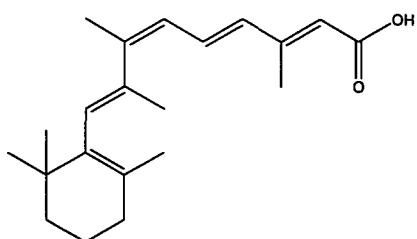
Alitreinoin
