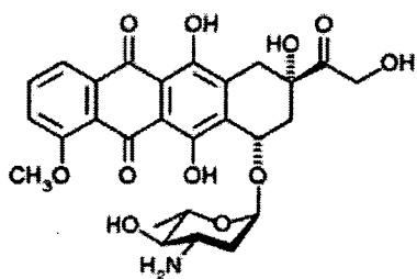
Epirubicin
