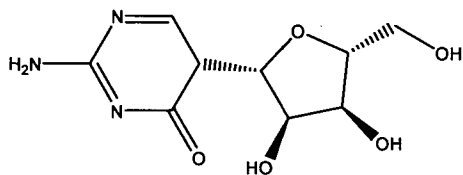
5-Azacytidine
