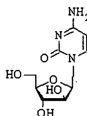
Cytarabine
