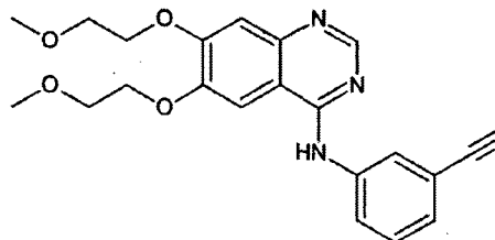
Erlotinib
