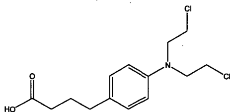
Chlorambucil
