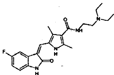
Sunitinib
