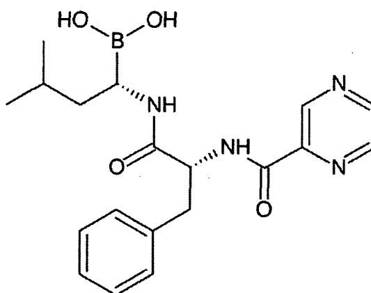
Bortezomib
