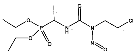
Fotemustine
