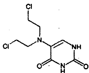
Uramustine
