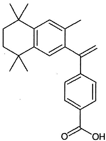
Bexarotene
