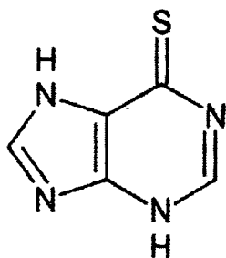
Mercaptopurine
