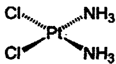
Cisplatin
