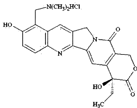
Topotecan
