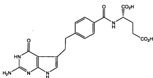
Pemetrexed
