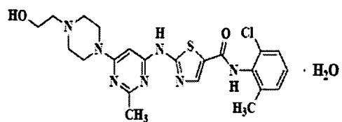
Dasatinib
