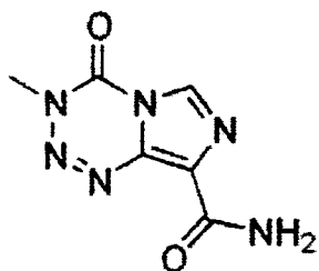
Temozolomide
