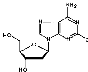
Cladribine
