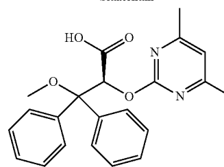
Ambrisentan
