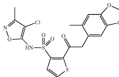
Sitaxentan
