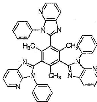
EB-4: E_a=2.1 , I_p=5.4
