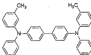
TPD : Ea=2.3, Ip=5.5
