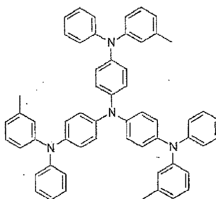
m-MTDATA : Ea=1.9, Ip=5.1
