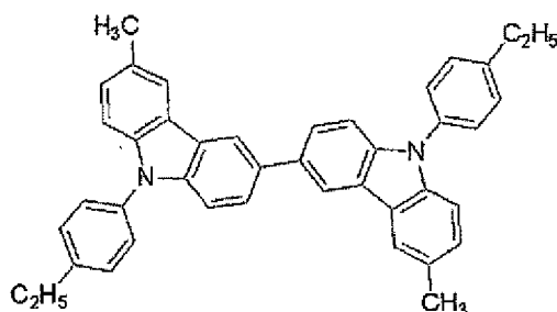
EB-5 : Ea=2.1, Ip=5.8
