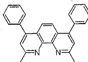
BCP: E_a=3.2 , I_p=6.7
