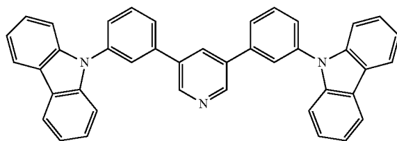
3,5DCzPPy
