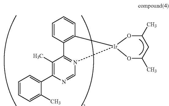
(xii) Ir(mpmpm) 2 (acac)
