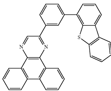
2mDBTPDBq-II
