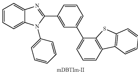
mDBTIm-II
