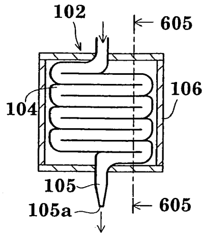
Fig.3B(PRIOR ART)
