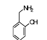
Salicylamine (SA)
