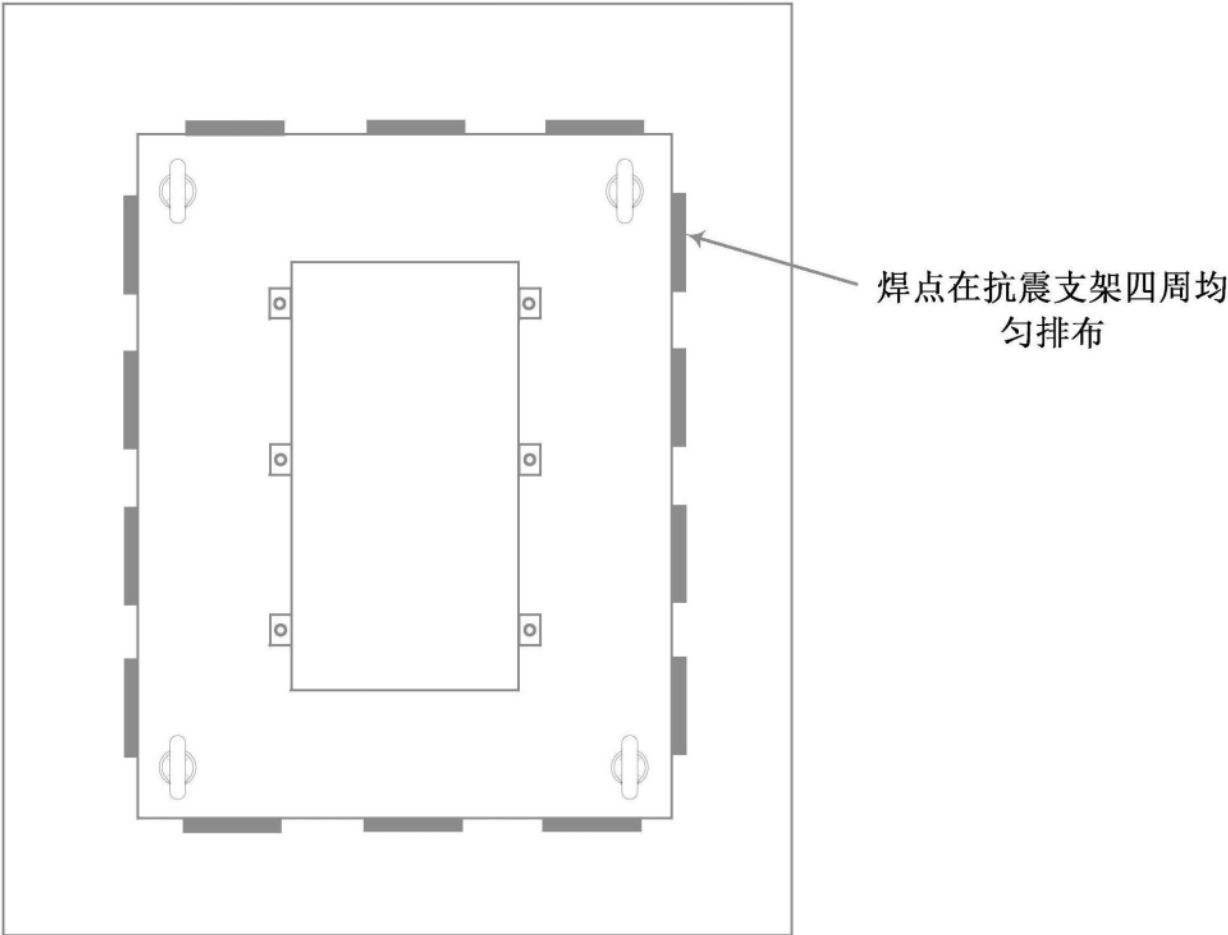
顶视图
