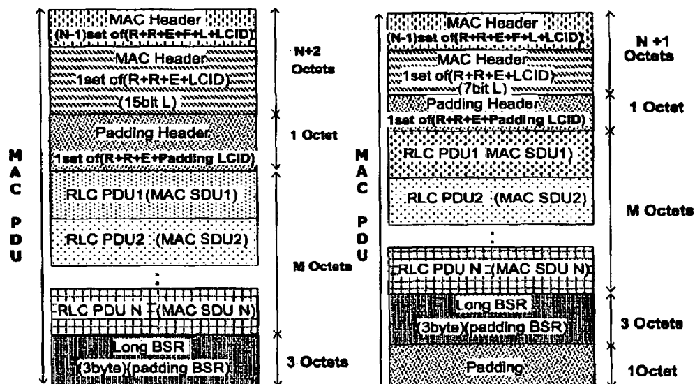
(b) case 2, implicit padding BSR
