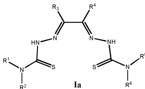
Chelatbildner
