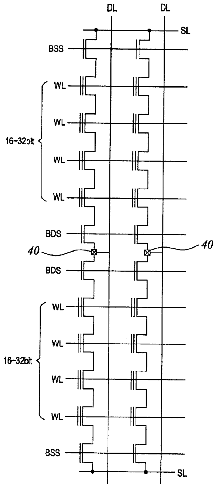
NAND Fig. 43
