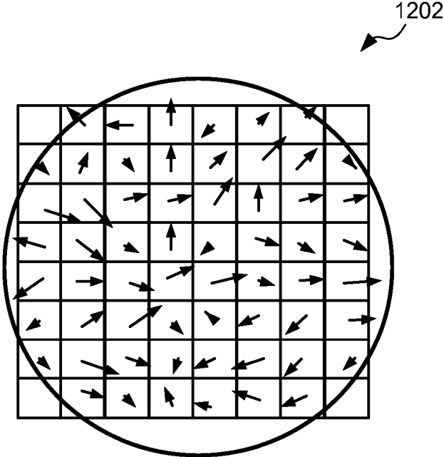
IMAGE GRADIENTS
