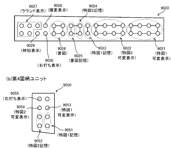
(a)特図LED基板
