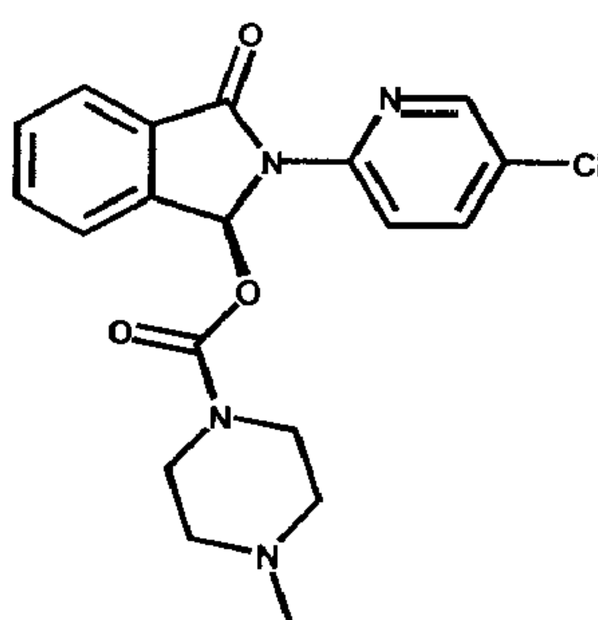
Eszopiclone
