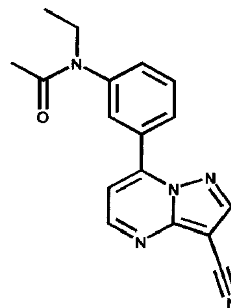
Zaleplon
