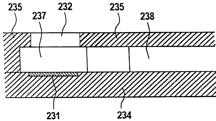
FIG. 64B
