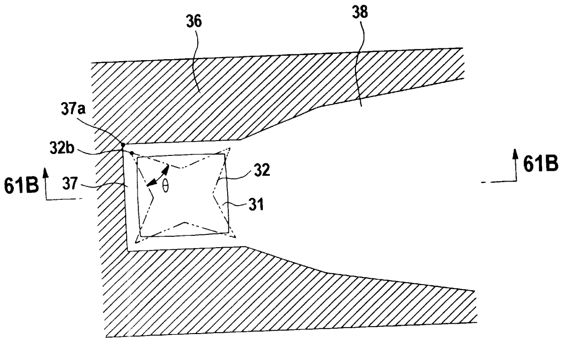
FIG. 61A
