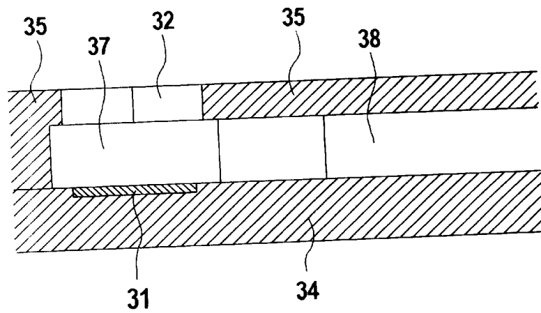
FIG. 61B
