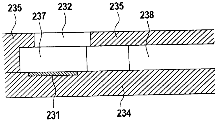
FIG. 62B
