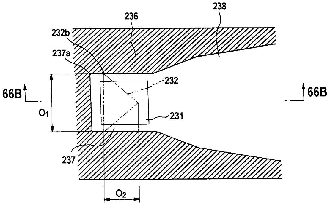
FIG. 66A
