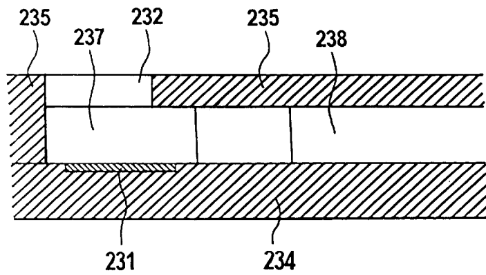
FIG. 65B
