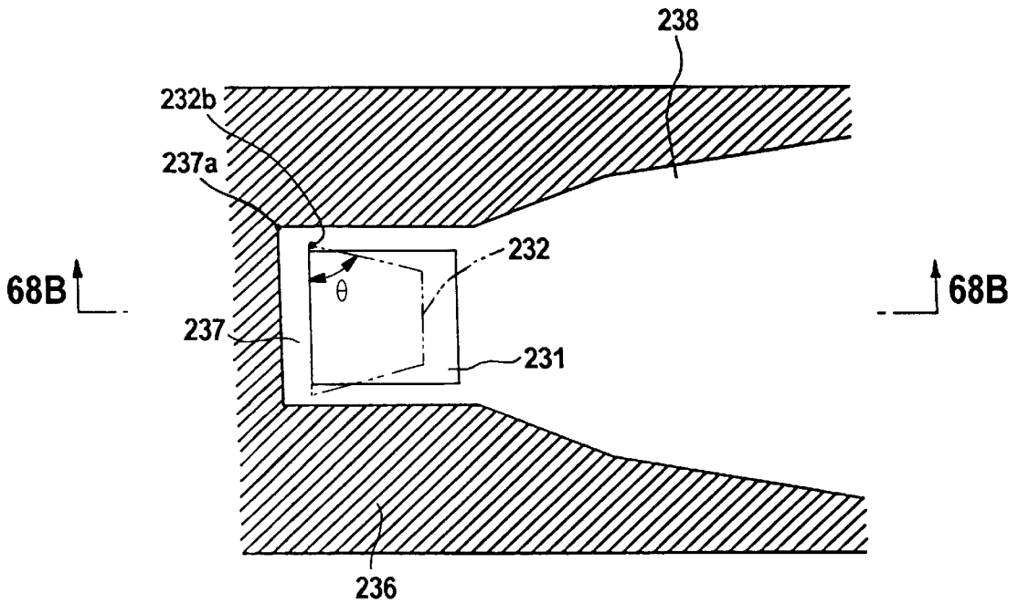
FIG. 68A
