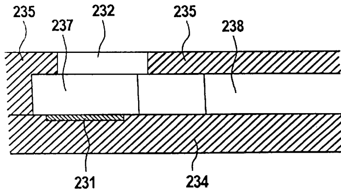
FIG. 67B
