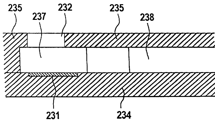
FIG. 68B
