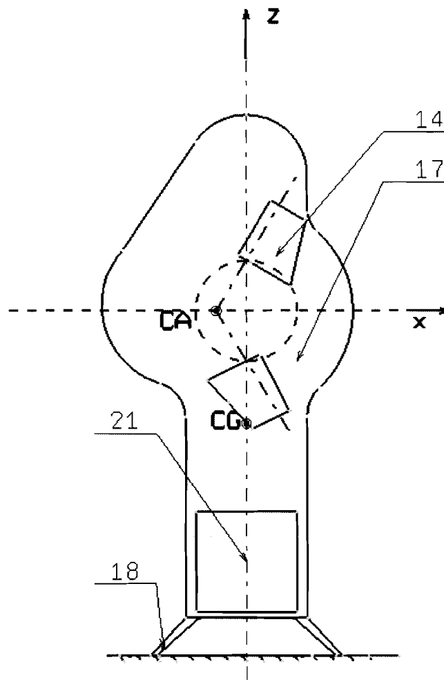
Fig. 3 Vedere laterala (stanga) a MAV ; CA-centru aerodinamic/focar al rotoarelor ; CG-centru de greutate (schita de principiu)
