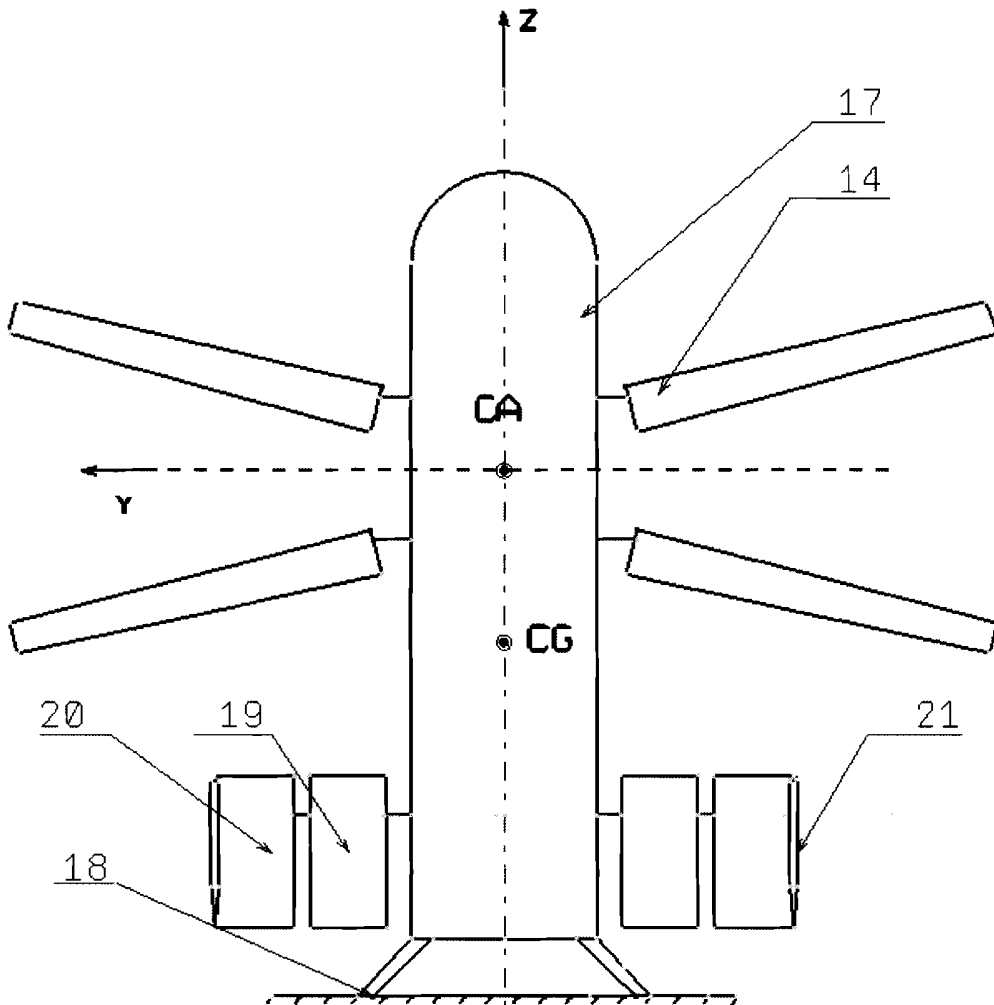
Fig. 2 Vedere frontala a MAV (schita de principiu)
