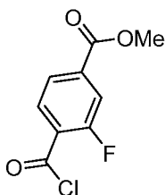
methyl 4-(chlorocarbonyl)-3-fluorobenzoate
