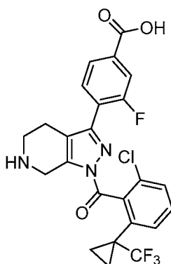
Example 20A
