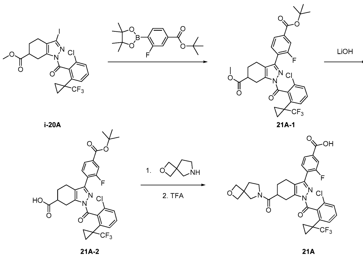
Example 21A
