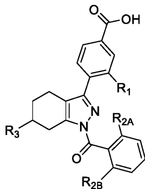
(I-1A)
