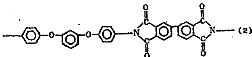
Chemische Formel 2
