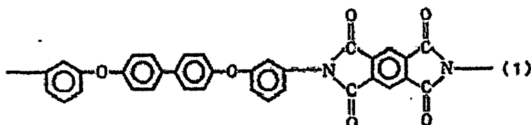
Chemische Formel 1
