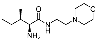
(2S,3R)-2-amino-3-methyl-N-(2-morpholinoethyl)pentanamide
