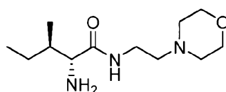
(2R,3R)-2-amino-3-methyl-N-(2-morpholinoethyl)pentanamide
