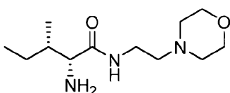
(2R,3S)-2-amino-3-methyl-N-(2-morpholinoethyl)pentanamide
