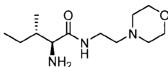
(2S,3S)-2-amino-3-methyl-N-(2-morpholinoethyl)pentanamide
