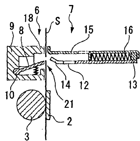
FIG.3F
