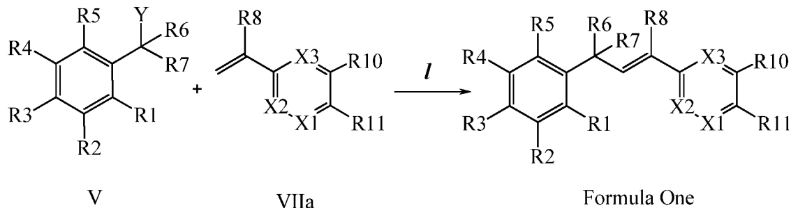
Scheme VI
