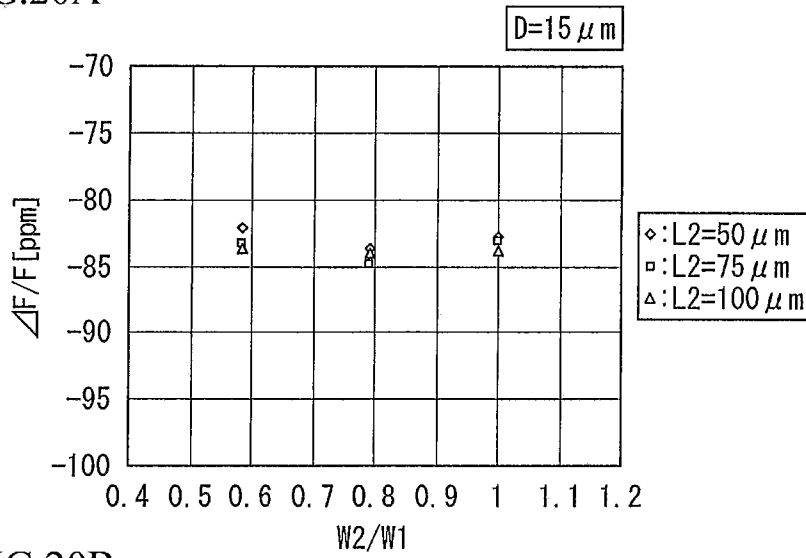
FIG.20B
