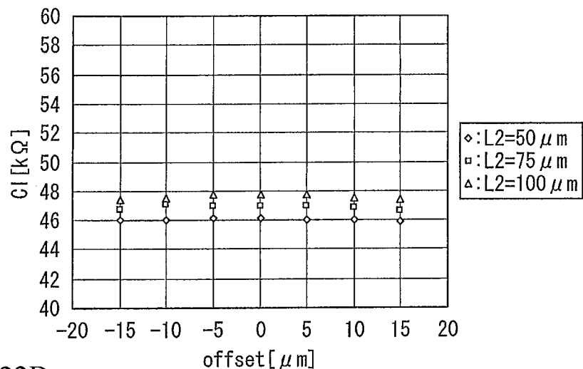
FIG.22B
