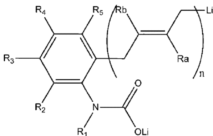
[Formule 1]
