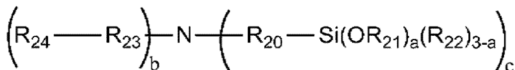
[Formule 2]
