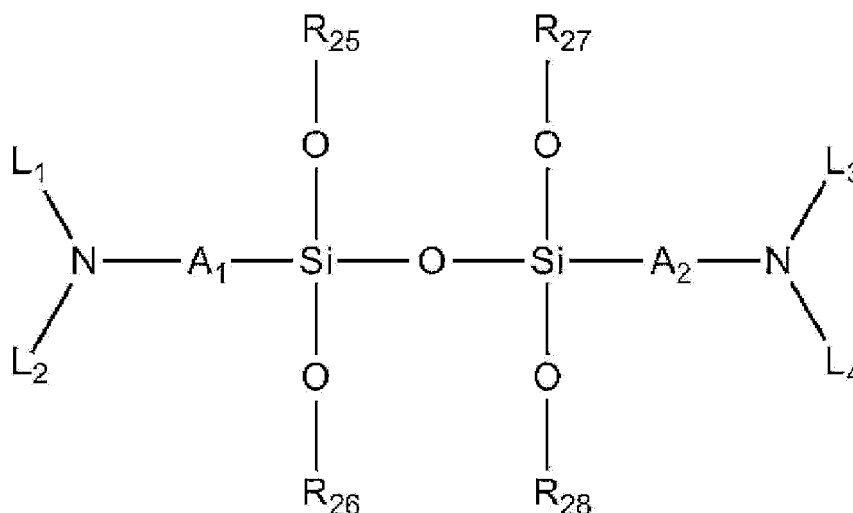
[Formula 3]
