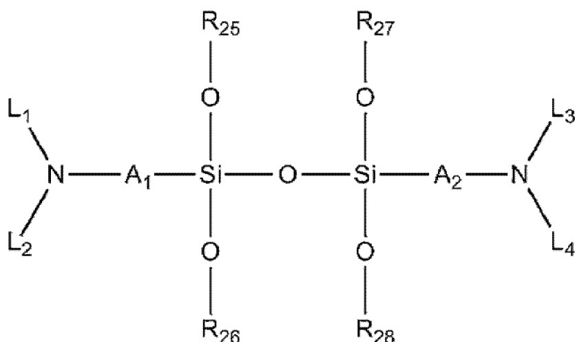
[Formule 3]
