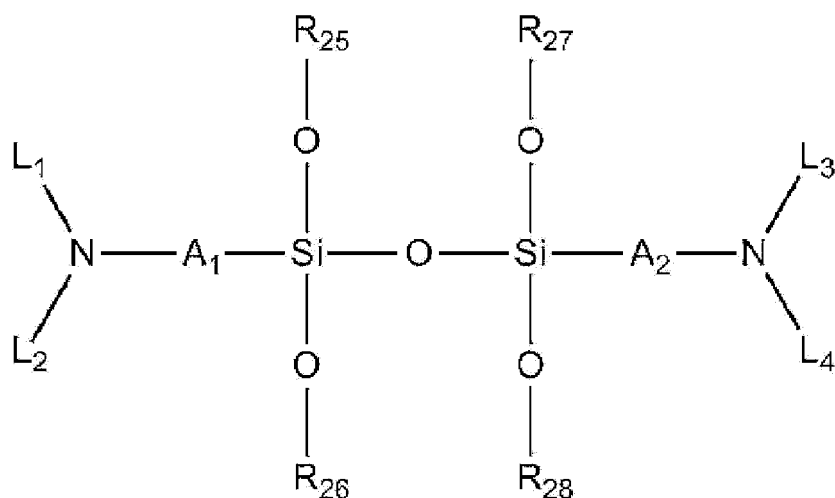
[Formula 3]
