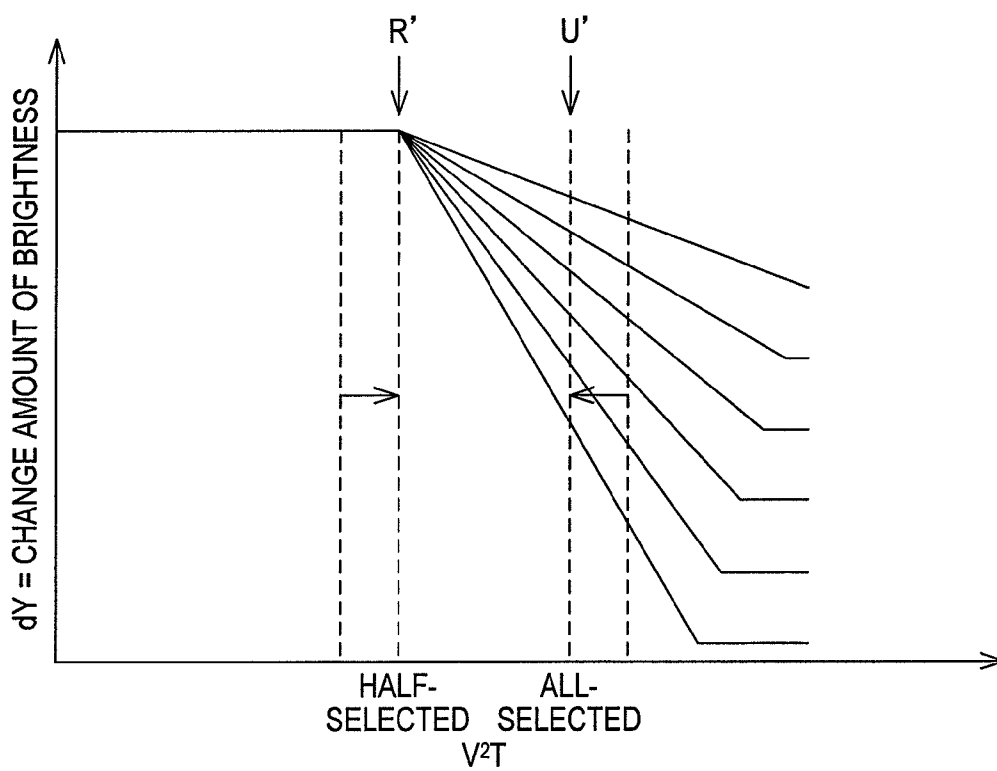
FIG.19B
