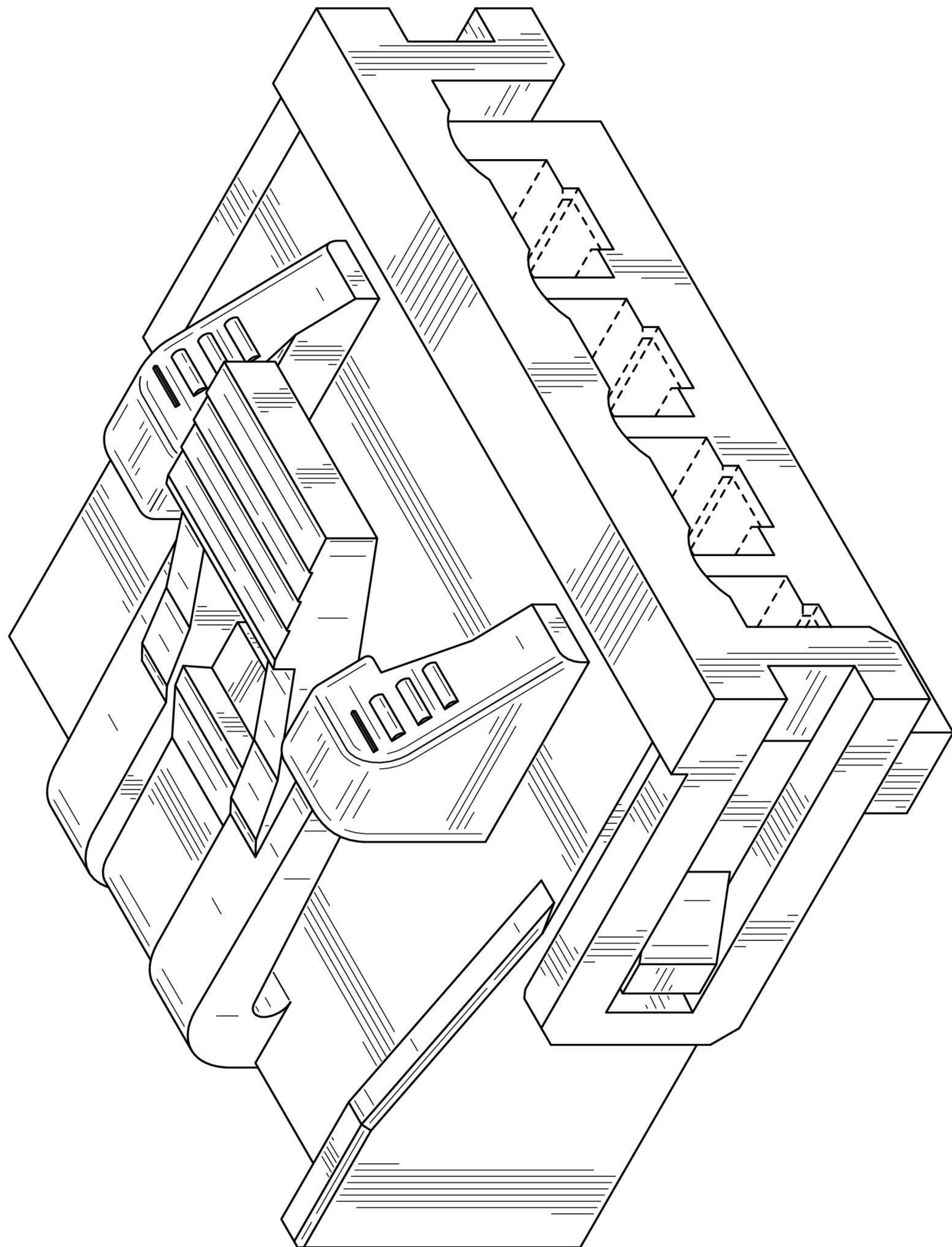
【前立體圖2】
