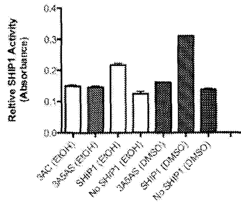
3 \alpha -Amino-5 \alpha -androstane (3A5AS)
