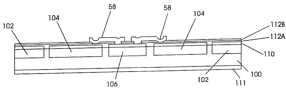
FIG. 3B
