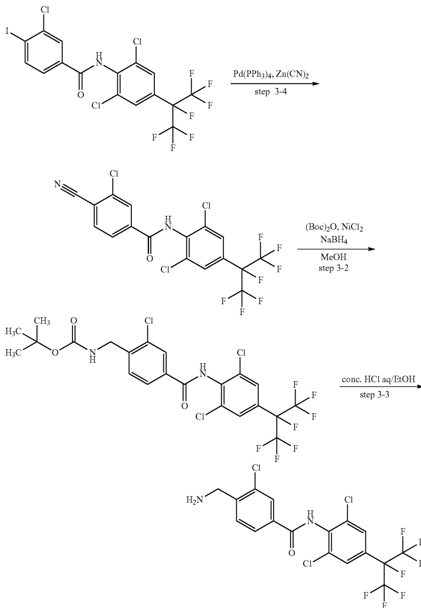
Scheme 3-1:
