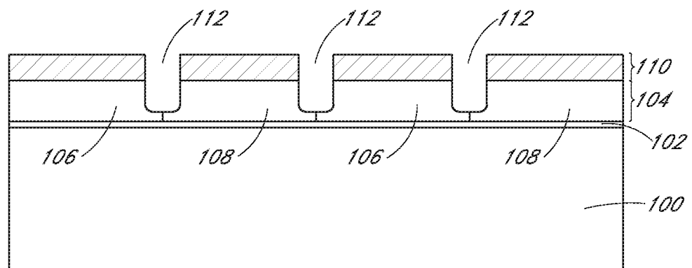
FIG. 1C(iv)
