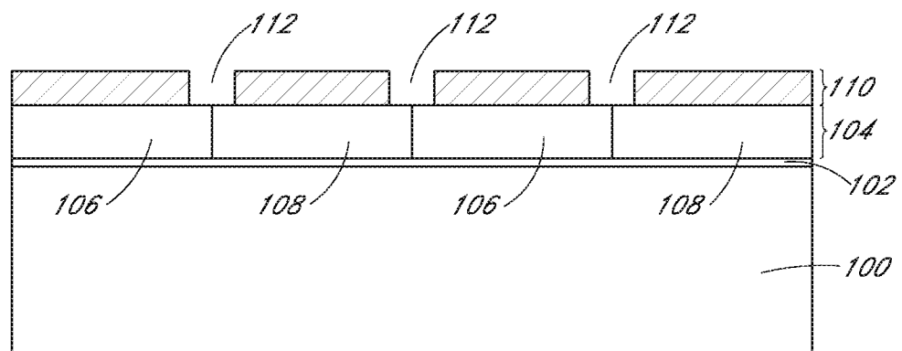
FIG. 1C(iii)
