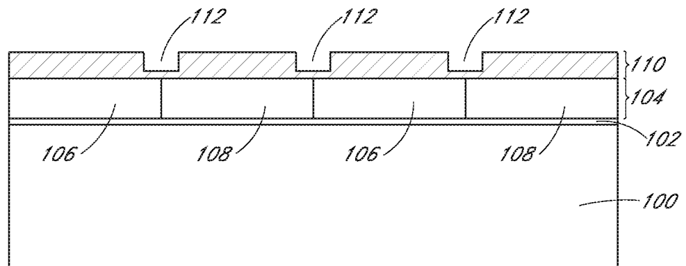
FIG. 1C(ii)
