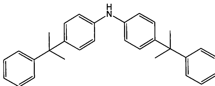
bis(4-(2-phenylpropan-2-yl)phenyl)amine
