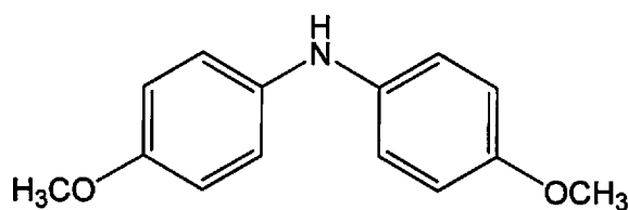
bis(4-methoxyphenyl)amine
