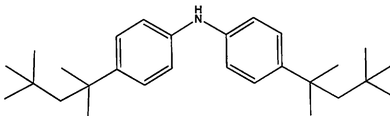
bis(4-(2,4,4-trimethylpentan-2-yl)phenyl)amine
