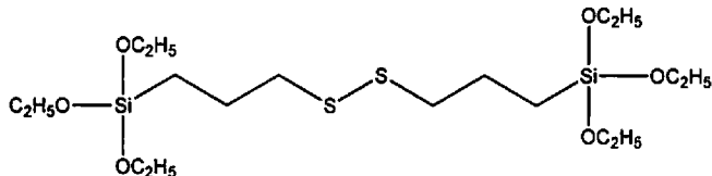
4,4,13,13-tetraethoxy-3,14-dioxa-8,9-dithia-4,13-disilahexadecane
