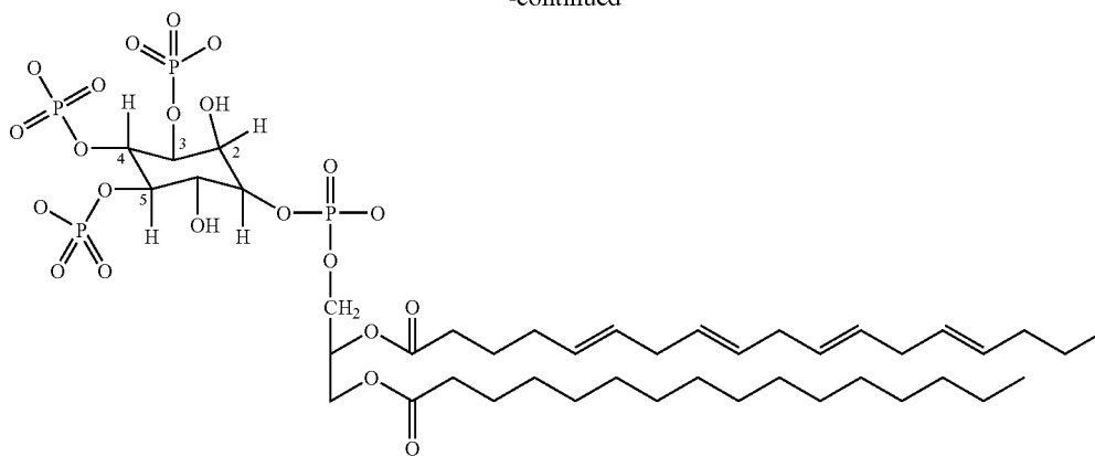
PtdIns(3,4,5)P 3
