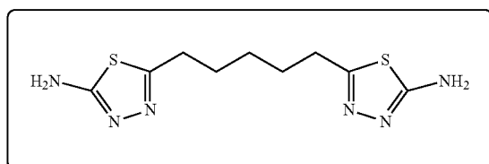
5,5'-(pentane-1,5-diyl)bis(1,3,4-thiadiazol-2-amine) (I-50)
