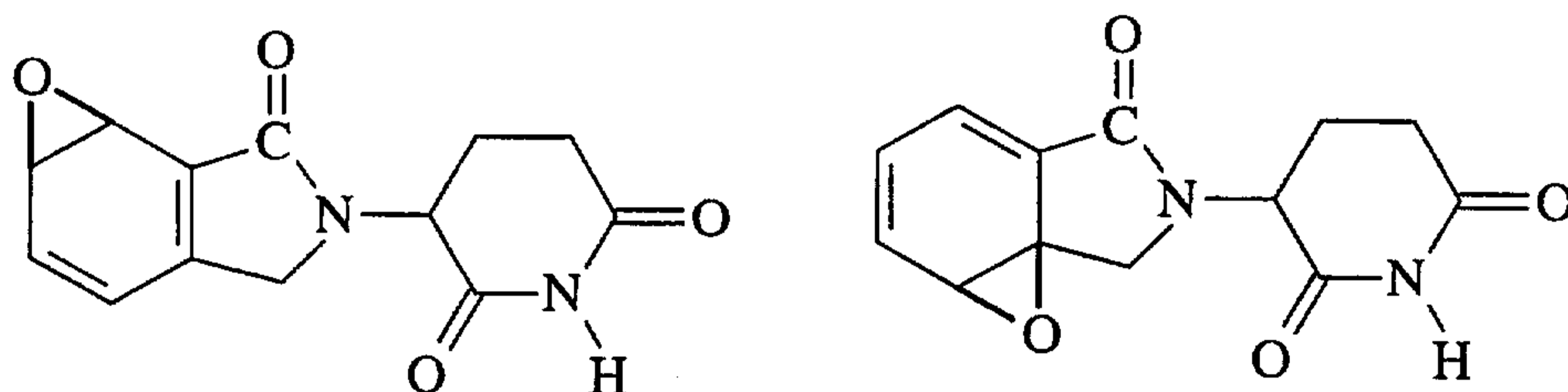
Epoxides of EM 12
