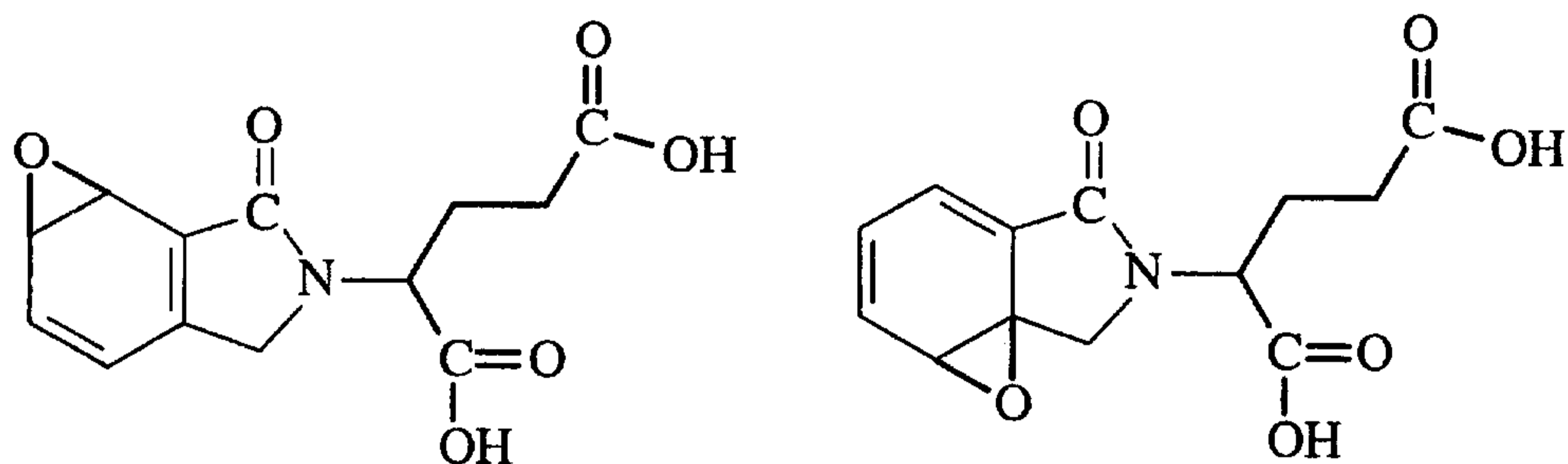
Epoxides of EM 138
