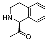
L-Tiq
