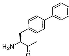
L-Bip
