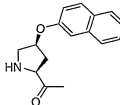
cis-Hyp(2-Naphthyl)
