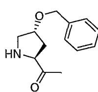
trans-Hyp(Bzl)
