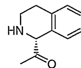
D-Tiq
