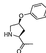
cis-Hyp(Phenyl)
