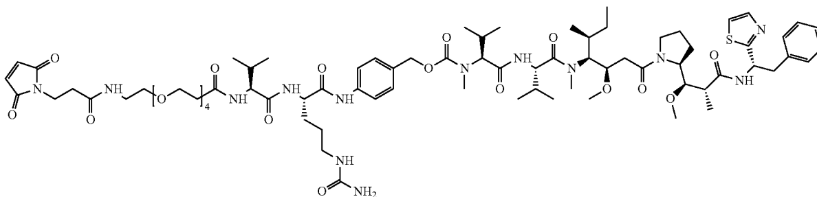
vc-MMAD:
