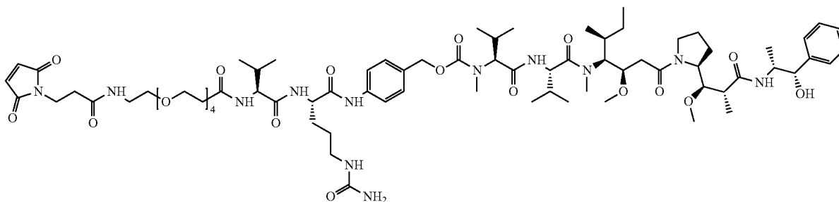
vc-MMAE:
