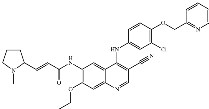
(E)-N-[4-[[3-Chloro-4-(2-pyridylmethoxy)phenyl]amino]-3-cyano-7-ethoxy-6-quinolyl]-3-(1-methylpyrrolidin-2-yl)prop-2-enamide
