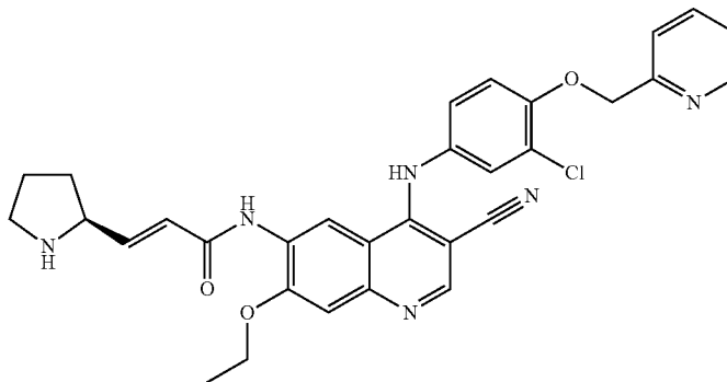
(E)-N-[4-[[3-Chloro-4-(2-pyridylmethoxy)phenyl]amino]-3-cyano-7-ethoxy-6-quinolyl]-3-[(2S)-pyrrolidin-2-yl]prop-2-enamide
