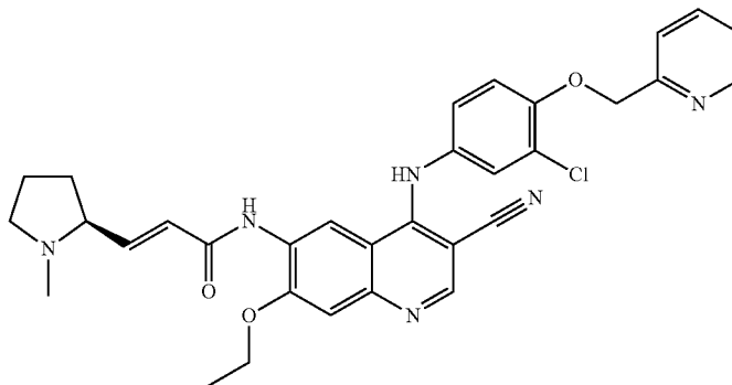
(E)-N-[4-[[3-Chloro-4-(2-pyridylmethoxy)phenyl]amino]-3-cyano-7-ethoxy-6-quinolyl]-3-[(2S)-1-methylpyrrolidin-2-yl]prop-2-enamide
