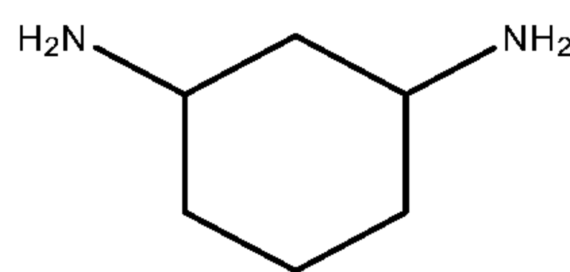
Cyclohexane-1,3-diamine,
