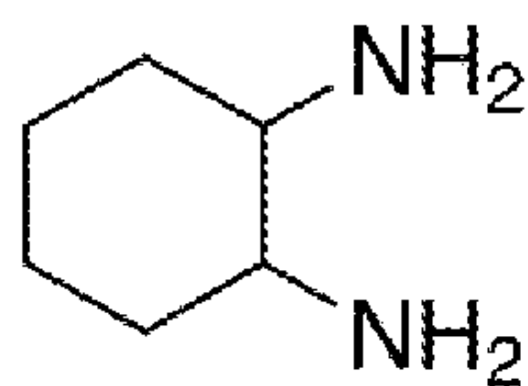
Cyclohexane-1,2-diamine
