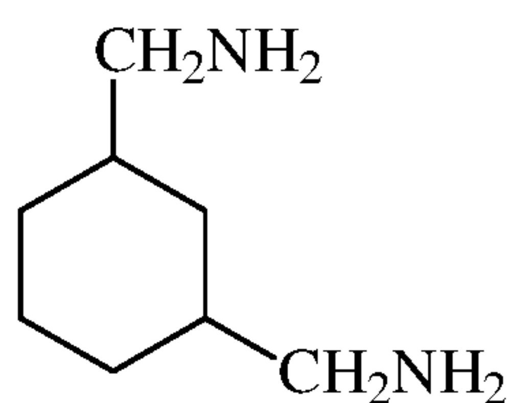
1, 3-bis(methylamine)-cyclohexane,
