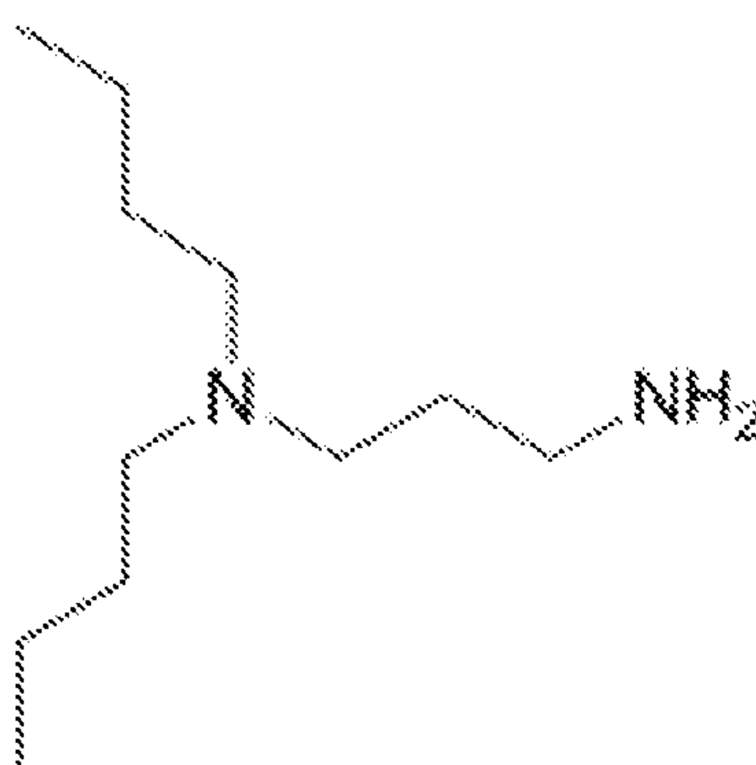
N,N' -dibutylpropane-1,3-diamine
