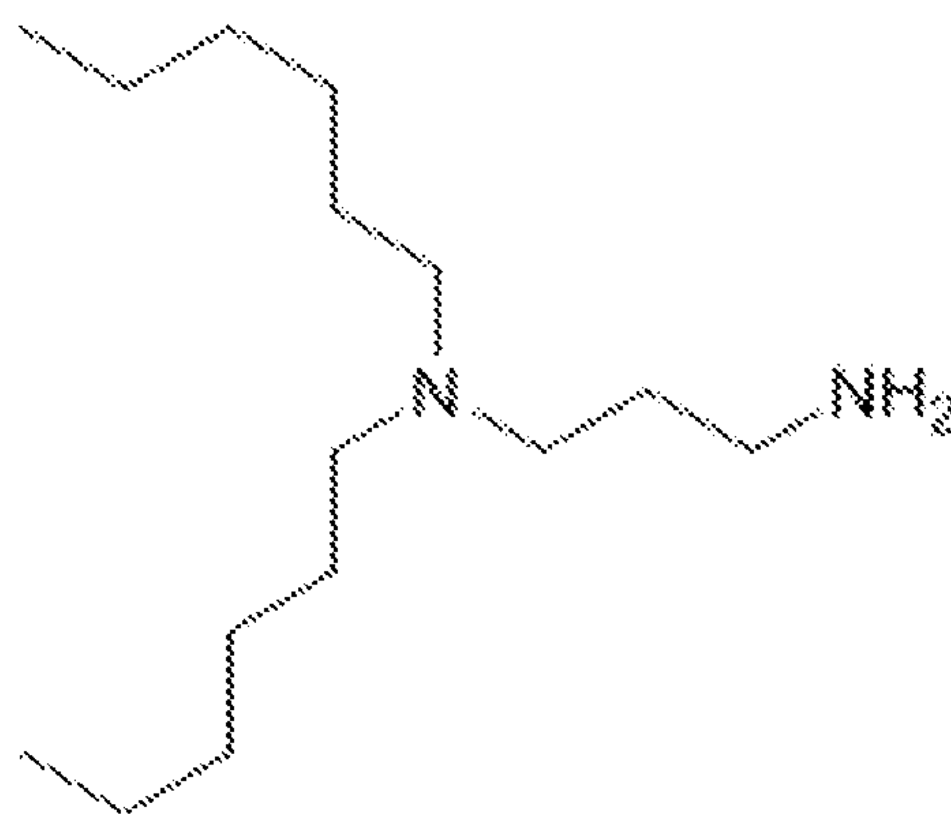
N,N' -dihexylpropane-1,3-diamine
