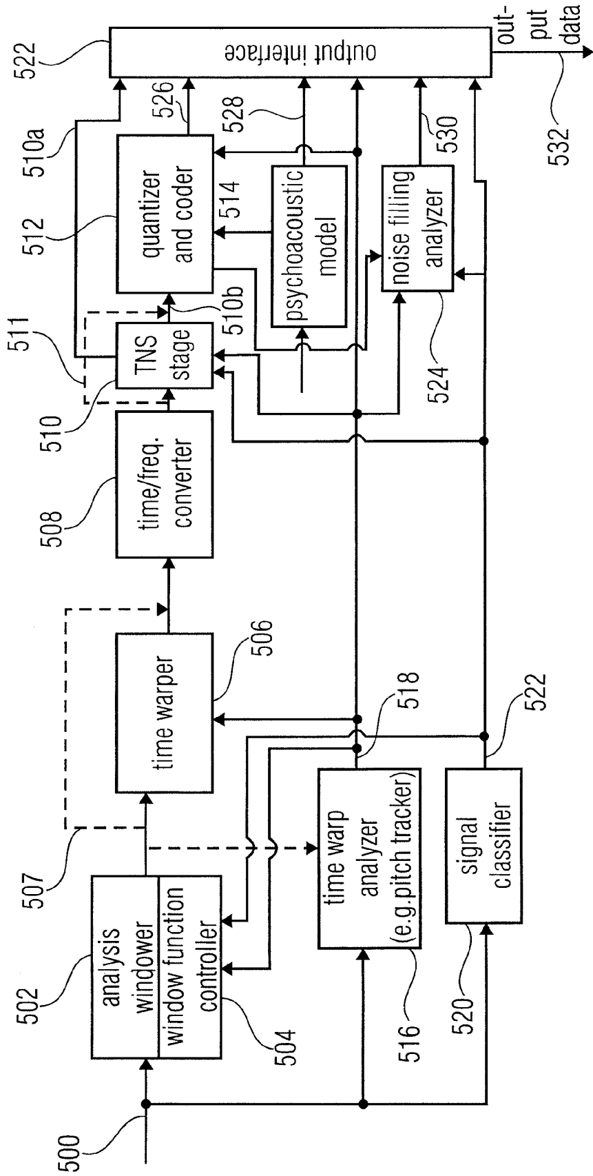
FIG 5A (ENCODER)
