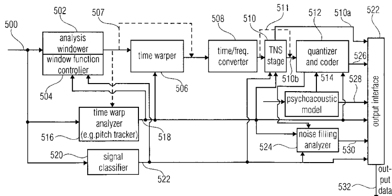
FIG 5A (ENCODER)
