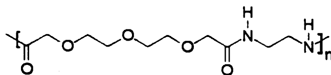
Polyoxaamides
